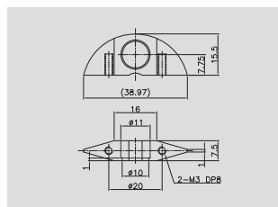
アルミブラケットC(半月型)
